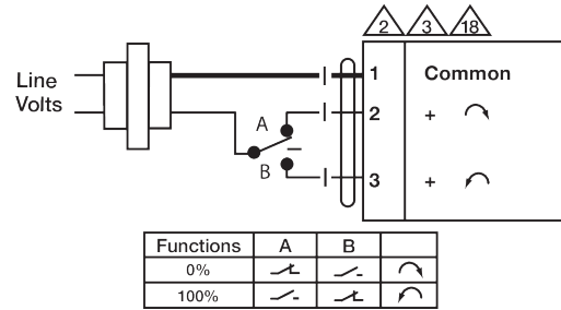
Transformador de ponto flutuante de 24 VCA
