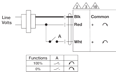
Transformador CA 24 V / CC 24 V 24 VCA
