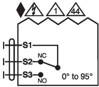
Interrupteurs auxiliaires
