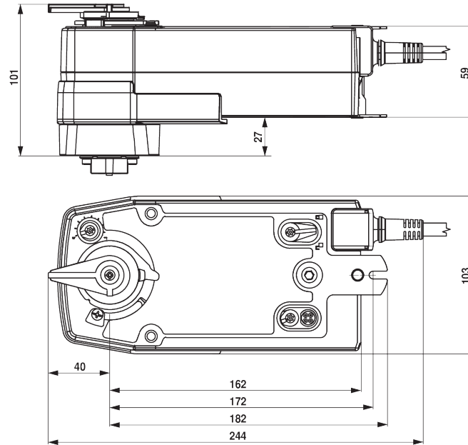
Méretjelölő ábrák
