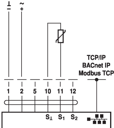
Collegamento contatto
