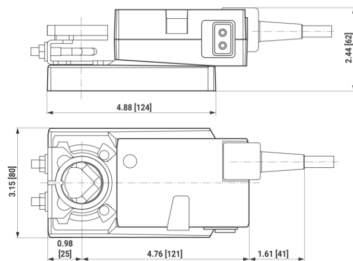
Desenhos dimensionais NMV-D3-MP
