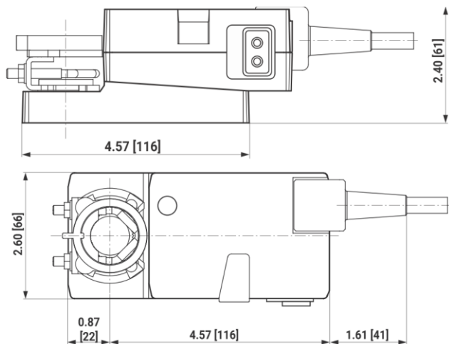
Desenhos dimensionais LHV-D3-MP
