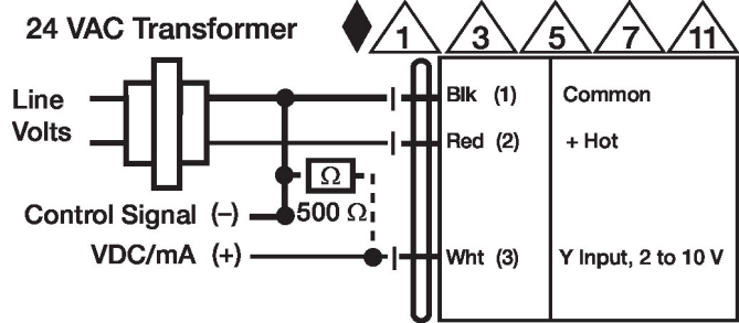
Esquema de conexionado Control 2...10 V / 4...20 mA
