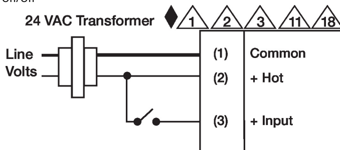
Esquema de conexión On/Off
