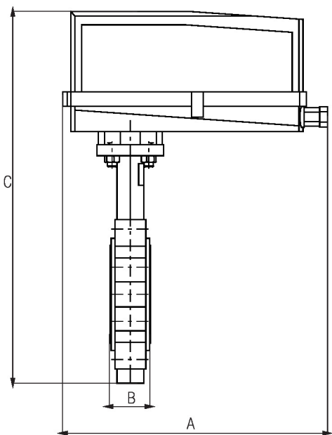
Válvula con actuador GRB..N4
