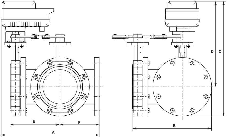
Válvula con actuador PK
