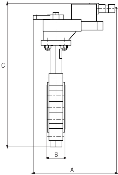
Válvula com atuador GRB(X)/GRCB(X)
