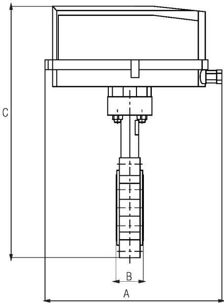
Válvula com atuador DKR..N4, DR..N4
