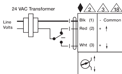
Ponto flutuante
