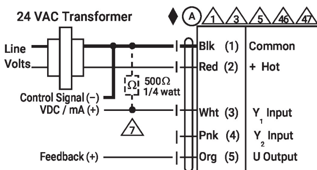
Controlo VDC / mA
