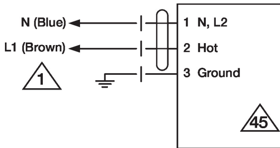
Cableado de control típico de compuerta de contención
