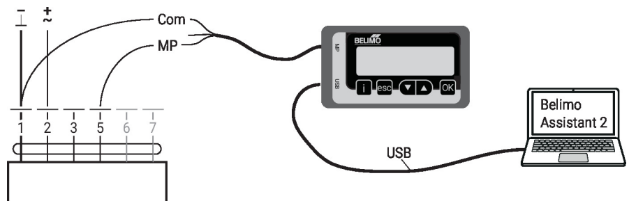
Conexión de Belimo Assistant 2
