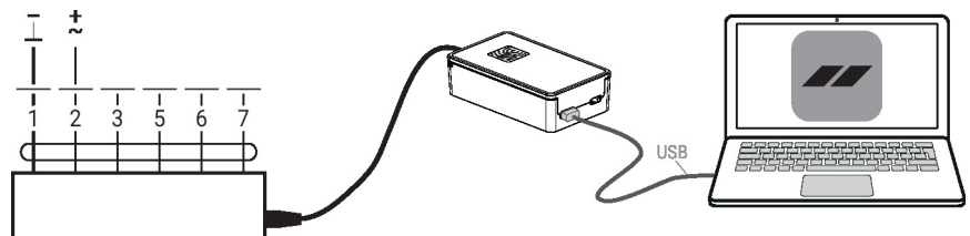
Conexión de Belimo Assistant 2
