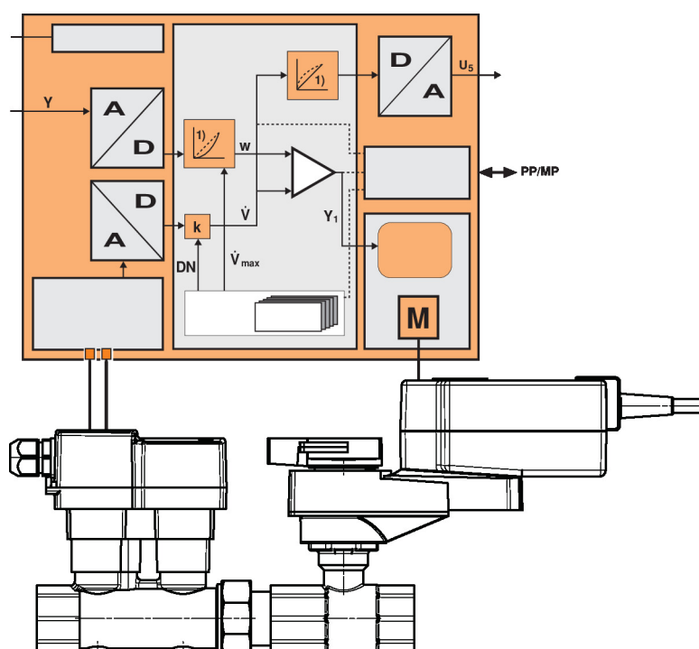
Schéma fonctionnel
