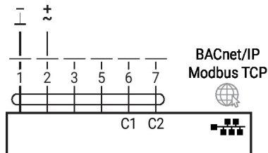
PoE avec BACnet/IP / Modbus TCP
