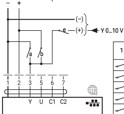
MP-Bus, alimentation par un raccordement à 3 fils
