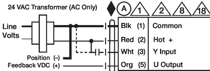
Commande PWM
