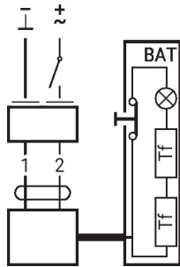
AC/DC 24 V, tout-ou-rien
