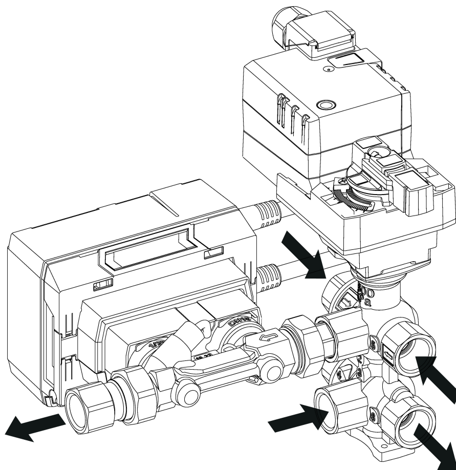
Capteur de débit dans le retour
