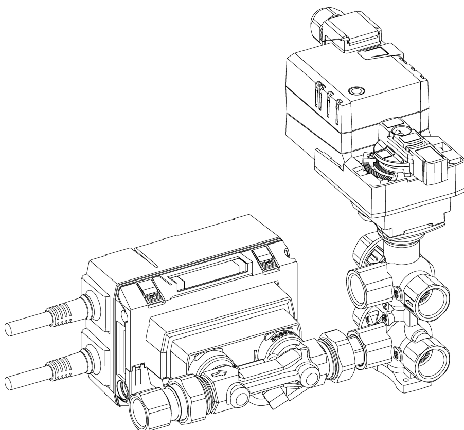
Capteur de débit dans le retour
