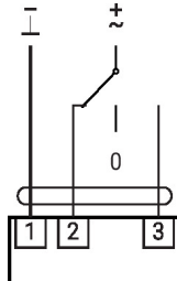
AC/DC 24 V, 3-punti
