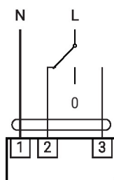
AC 230 V, 3-punti
