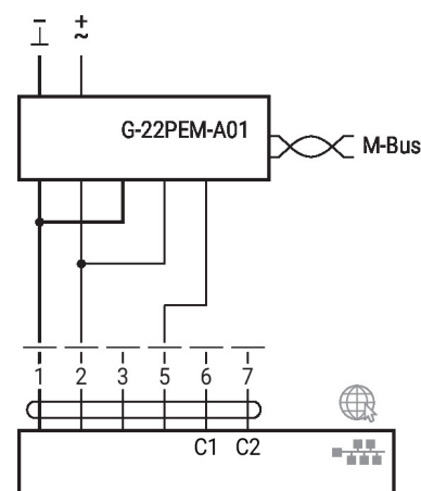
Szyna M-Bus z konwerterem w trybie równoległym z PoE z BACnet/IP / Modbus TCP
