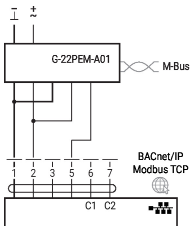
Szyna M-Bus z konwerterem w trybie równoległym z BACnet/IP / Modbus TCP
