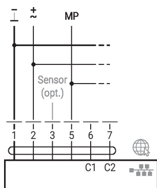
Szyna M-Bus z konwerterem w trybie równoległym z BACnet/IP / Modbus TCP
