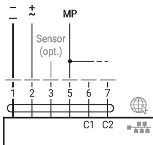
Szyna M-Bus z konwerterem w trybie równoległym z BACnet/IP / Modbus TCP
