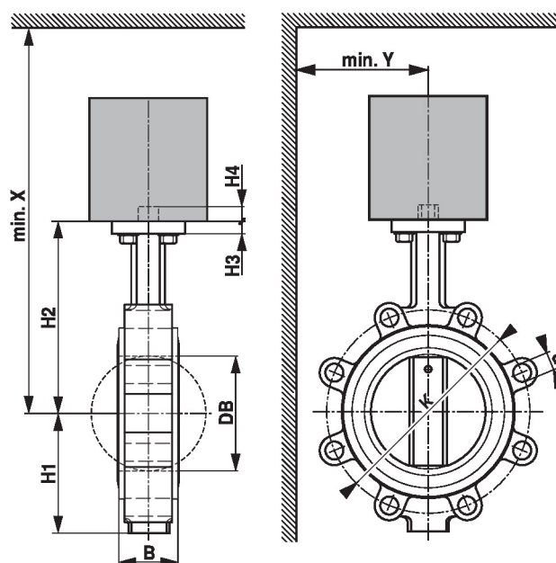
Måttritningar
