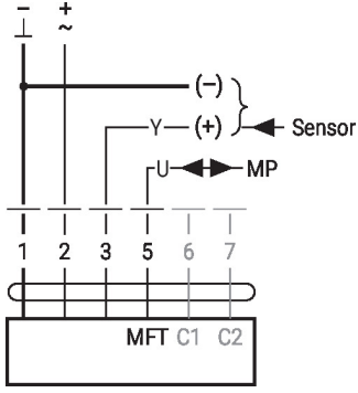
MP-Bus üzerinden çalışma
