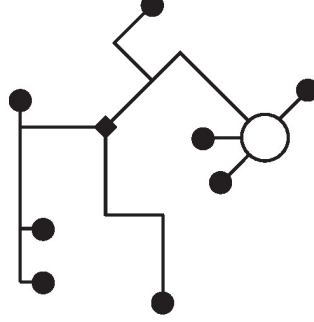
MP-Bus kablo topolojisi
