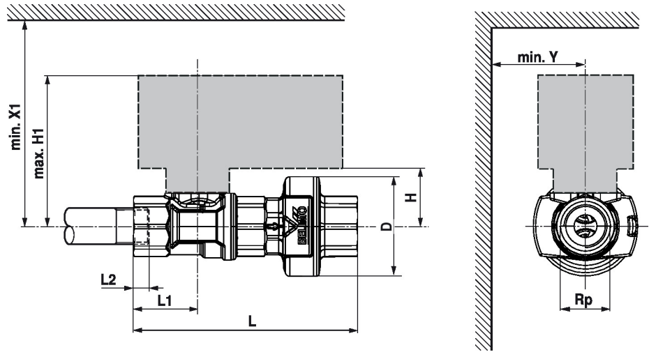
尺寸图
