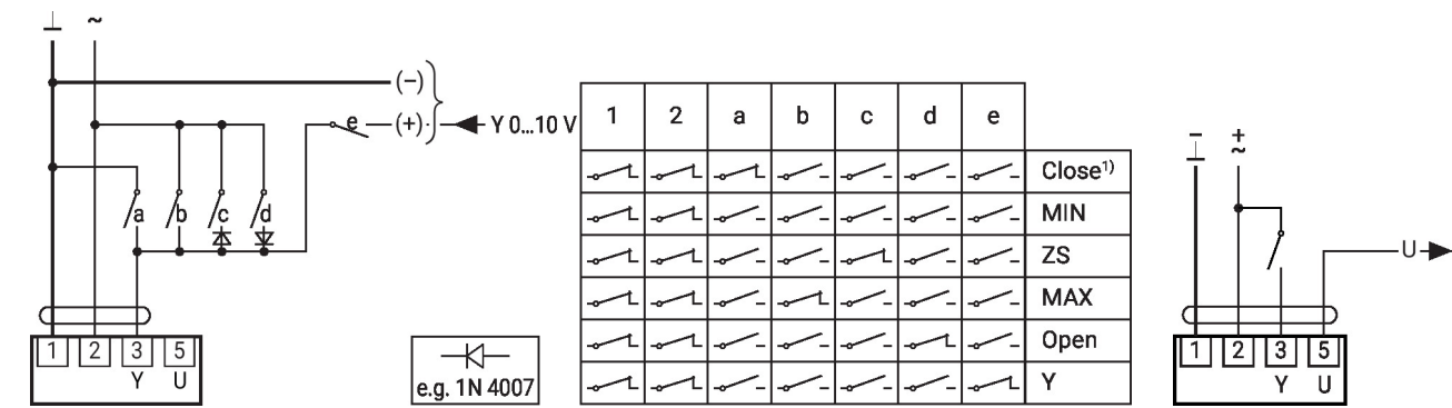
AC 24V继电器限位控制
