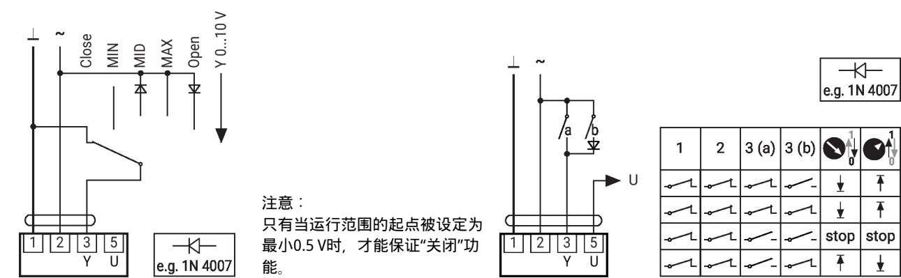
AC 24V旋转开关限位控制
