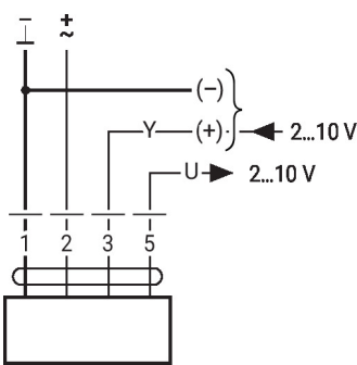
AC/DC 24 V, 调节型
