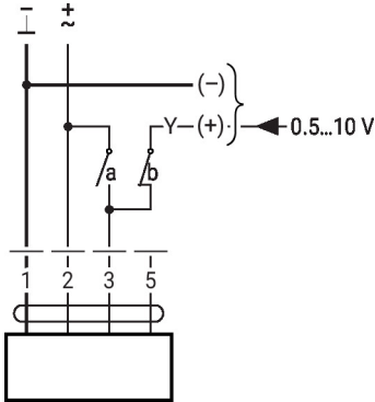
超驰控制 (防冻回路)
